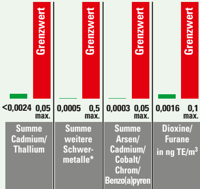
SIEDLUNGSABFALLVERBRENNUNGSANLAGE LINIE 2
