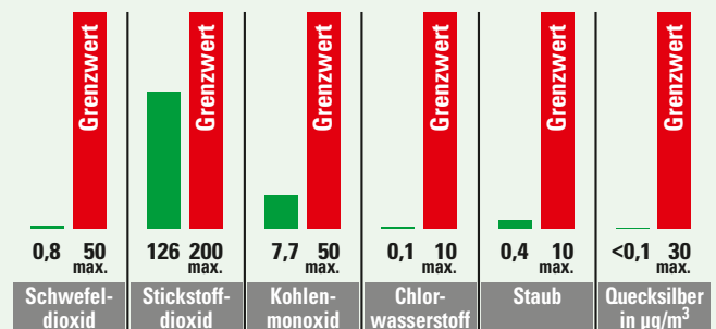
SIEDLUNGSABFALLVERBRENNUNGSANLAGE LINIE 4
