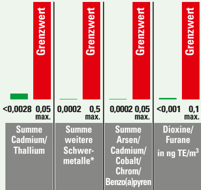
INDUSTRIEABFALLVERBRENNUNGSANLAGE LINIE 2
