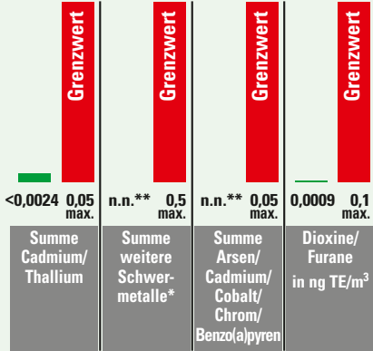
SIEDLUNGSABFALLVERBRENNUNGSANLAGE LINIE 4
