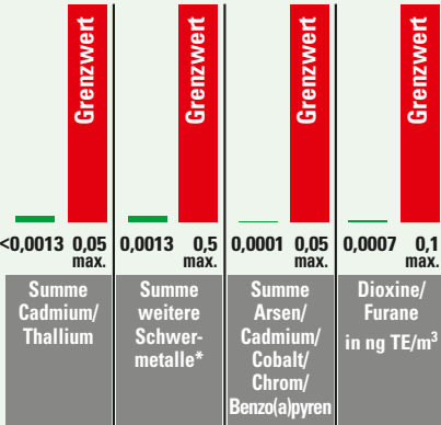
INDUSTRIEABFALLVERBRENNUNGSANLAGE LINIE 1
