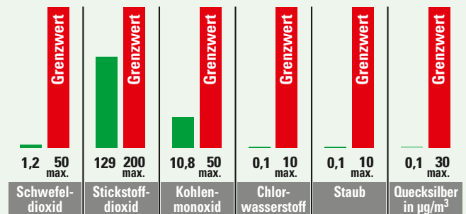
SIEDLUNGSABFALLVERBRENNUNGSANLAGE LINIE 2
