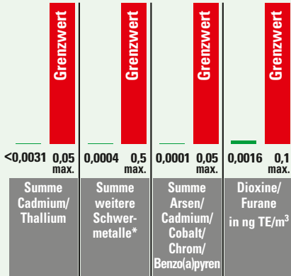
SIEDLUNGSABFALLVERBRENNUNGSANLAGE LINIE 1
